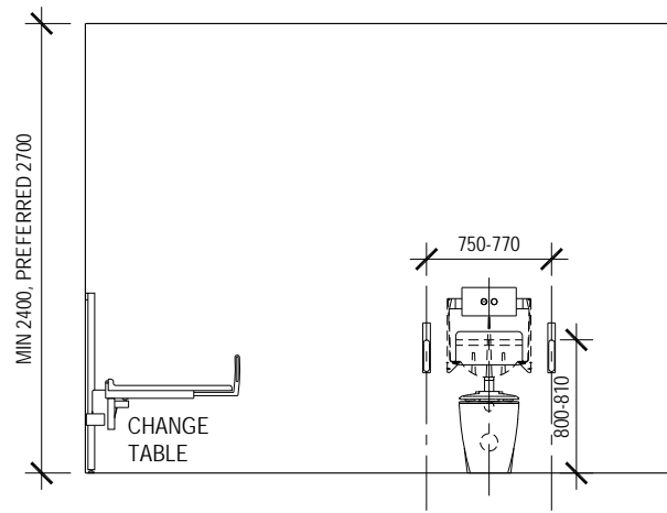
ELEVATION A
